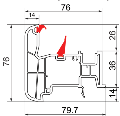
81/6 Krilo vrata Z (unutrašnje otvaranje)
