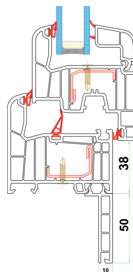
76/6 Štok 00490 Pervaz štoka Lajsna za staklo 24mm
