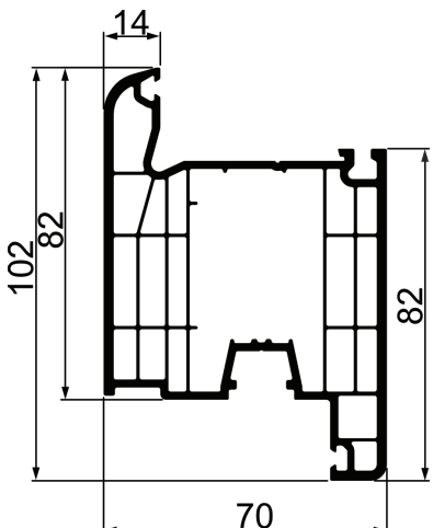
82/6 Krilo vrata Z (unutrašnje otvaranje)
