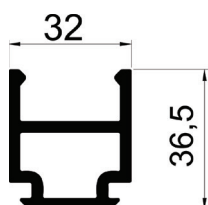
00112 Podprozorski profil
