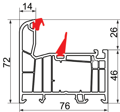
72/6 Štok (veliki)
