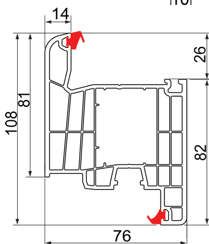
81/6 Krilo vrata Z (unutrašnje otvaranje)
