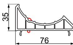
01573 (veliki) Adapter za cev
