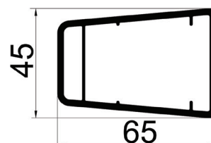
00117 Statičko ojačanje
