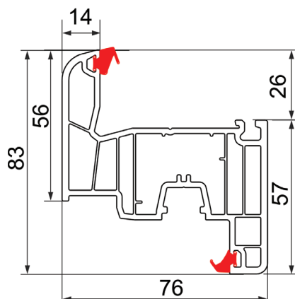
72/6 Štok (veliki)
