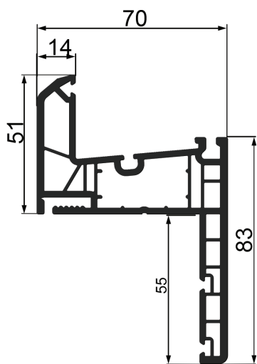
70 Renovacioni ram
