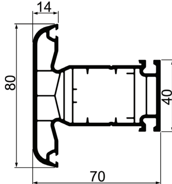
80/6 Prečka
