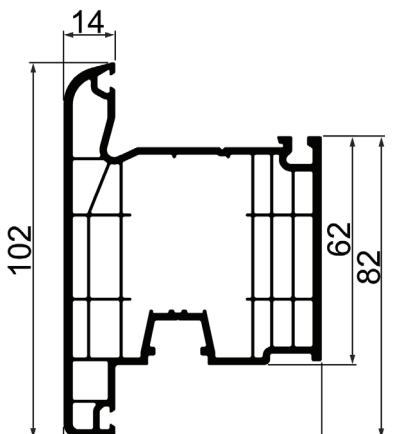
102/6 Krilo vrata T (spoljašnje otvaranje)
