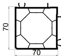
00088 Spojni profil 90°/70
