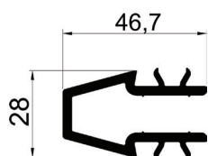
01566 Spojni profil
