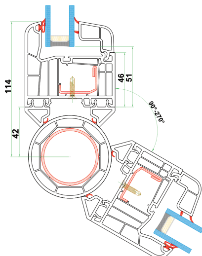
76/6 Štok 01551 Adapter za cev (mali) 6K.616 Spojni profil Lajsna za staklo 24mm
