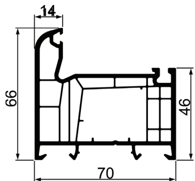
66/6 Štok (veliki)
