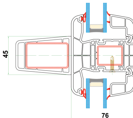
96/6 Prečka 00117 Statičko ojačanje 00490 Pervaz štoka Lajsna za staklo 24mm
