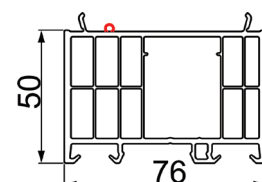
01554 Proširenje štoka 50
