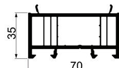
00100 Proširenje štoka 35
