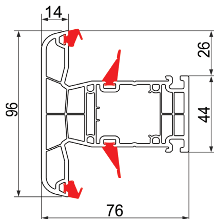
96/6 Prečka
