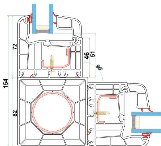
76/6 Štok 01550 Spojni profil 90°/82 Lajsna za staklo 24mm
