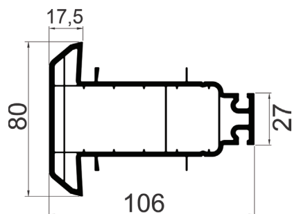
01567 Ojačani spojni profil
