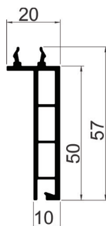
00490 Pervaz štoka
