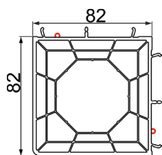
01550 Spojni profil 90°/82
