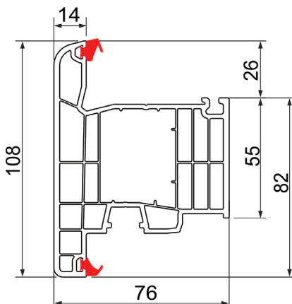
108/6 Krilo vrata T (spoljašnje otvaranje)
