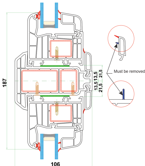
76/6 Štok 01567 Ojačani spojni profil Lajsna za staklo 24mm Lajsna za staklo 44mm
