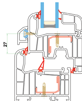
76/6 Štok 56/6 Krilo 00491 Okapnica krila Lajsna za staklo 24mm
