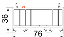
01553 Proširenje štoka 36
