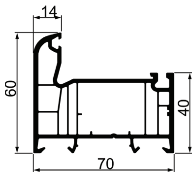
60/6 Štok (mali)
